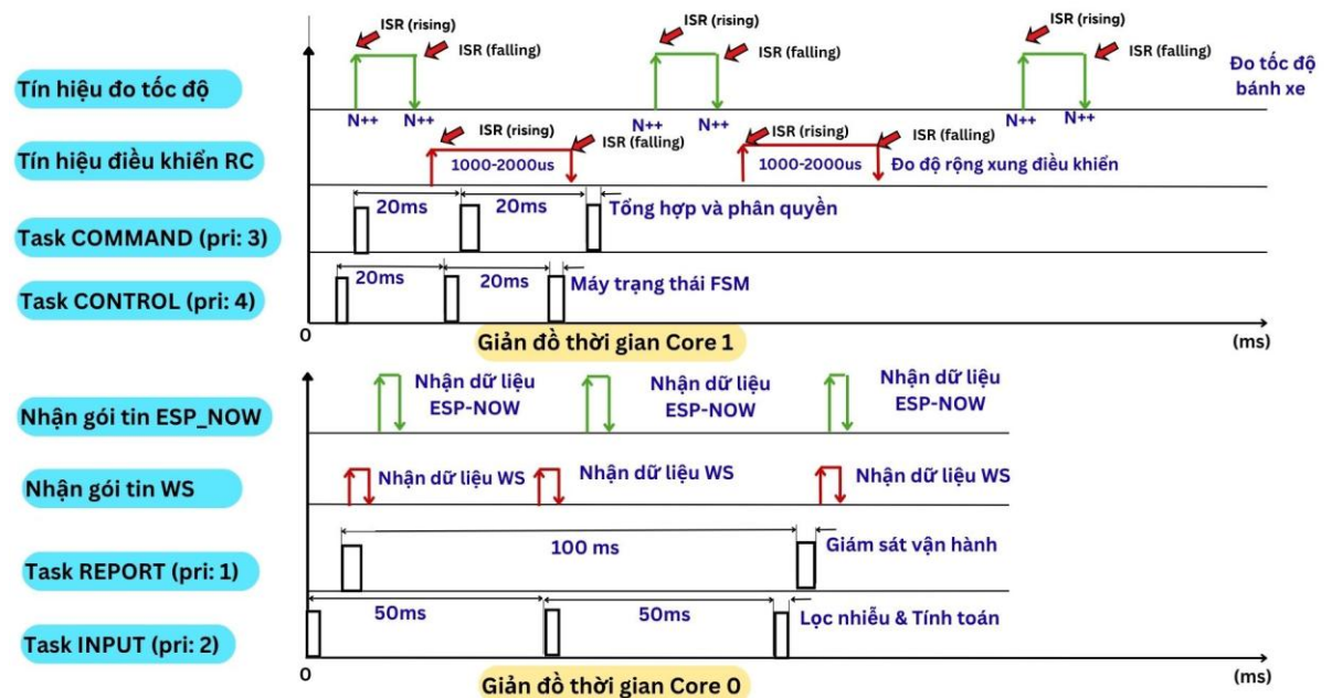
Hình 1.6.1. Giản đồ thời gian hoạt động các tác vụ
